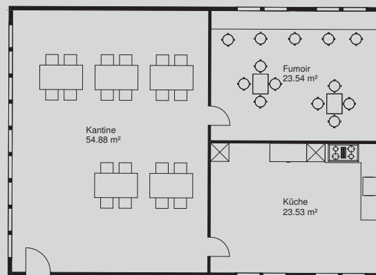
Abb.: Beispielgrundriss einer Kantine mit Küche und Fumoir Länge 12.01 m, Breite 8.58 m
